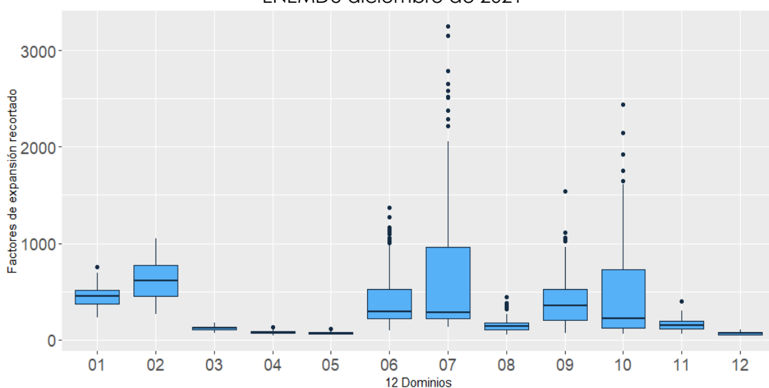
Gráfico 3. Diagramas de caja y bigote del factor de expansión recortados de la ENEMDU diciembre de 2021
